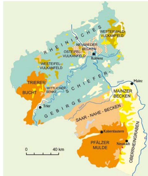
Geologisch-tektonische Grobseinheiten in Rheinland-Pfalz.
